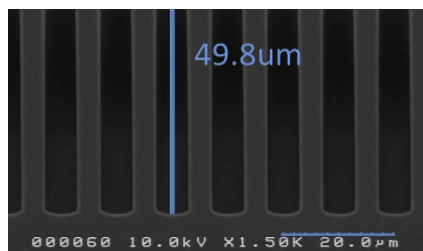
D-RIE(トレンチ)
