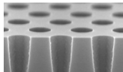
P-SiNホール
