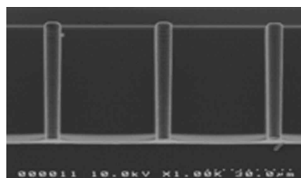
D-RIE(ピラー)
